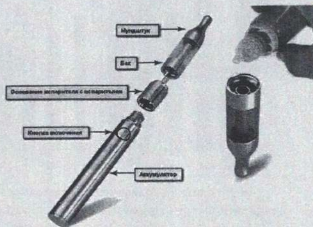
Рис. 3. Устройство электронной сигареты
